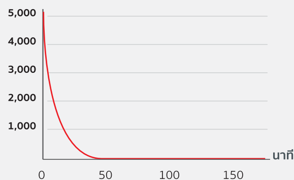
ปริมาณฝุ่น PM 0.1 (microgram/m 3 )
