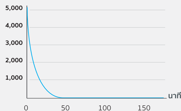
ปริมาณฝุ่น PM 2.5 (microgram/m 3 )
